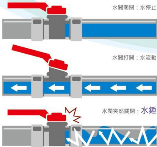
水錘示意圖
